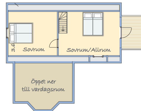
Loft (1:200)
