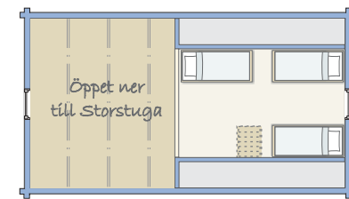
Lofet skala 1:200
